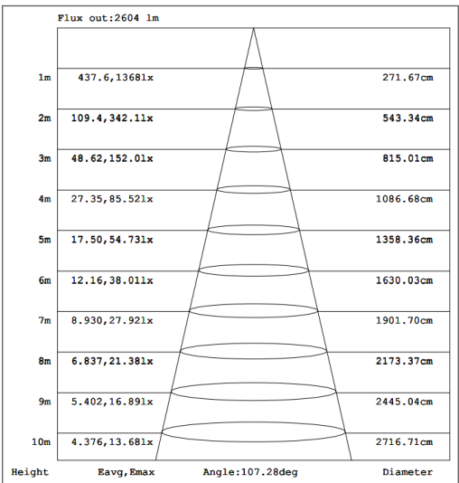
DIAGRAMA ILUMINACIÓN - DISTANCIA
