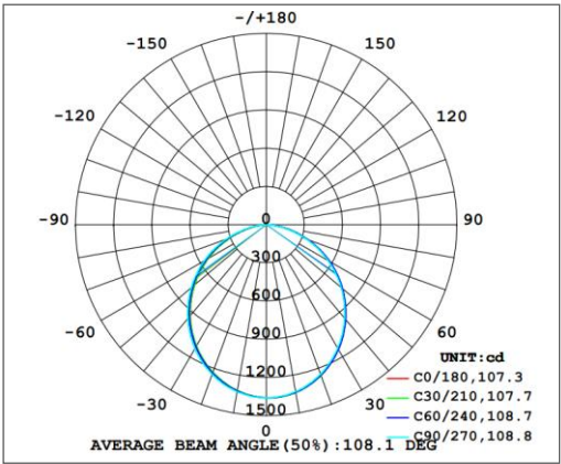
DIAGRAMA FOTOMÉTRICO
