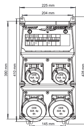
PLANO MECÁNICO
